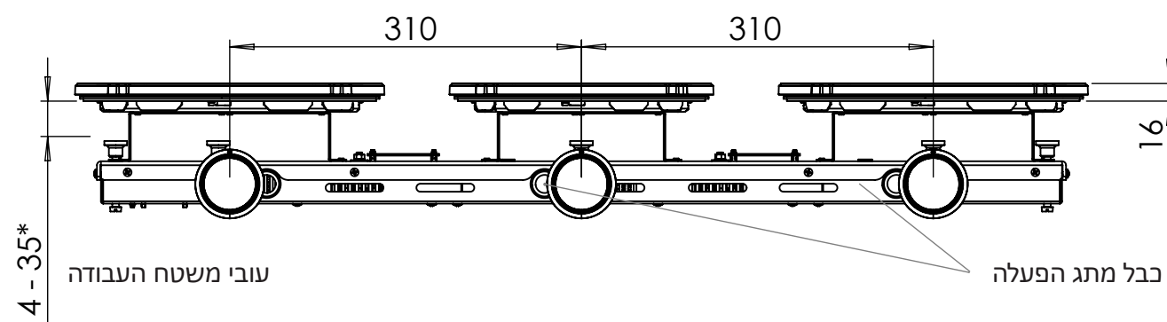
מבט חזיתי
