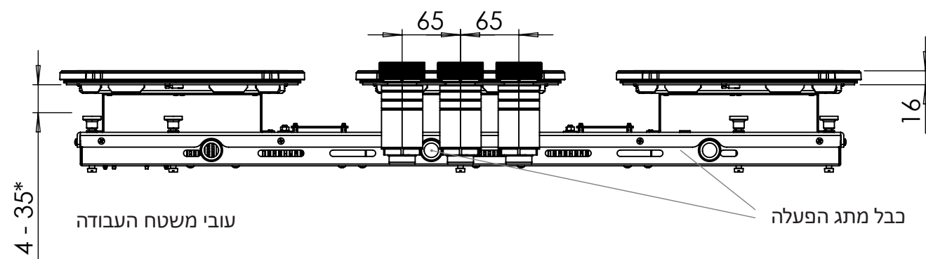
מבט חזיתי
